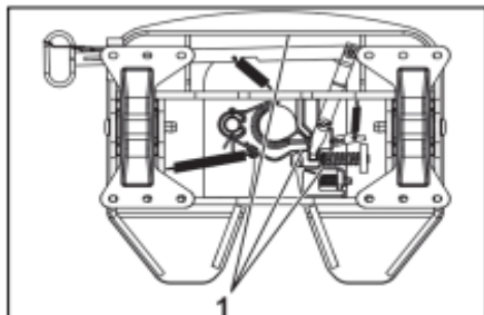
1. Khóa ngừng, pít tông, nệm và khóa trước
